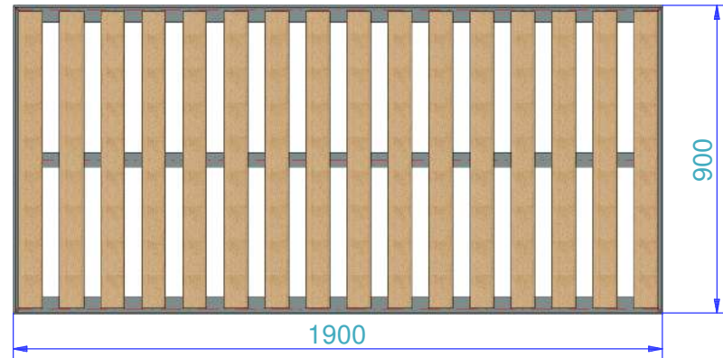
Einsatz mit Gitterrost zu Bett E190A
