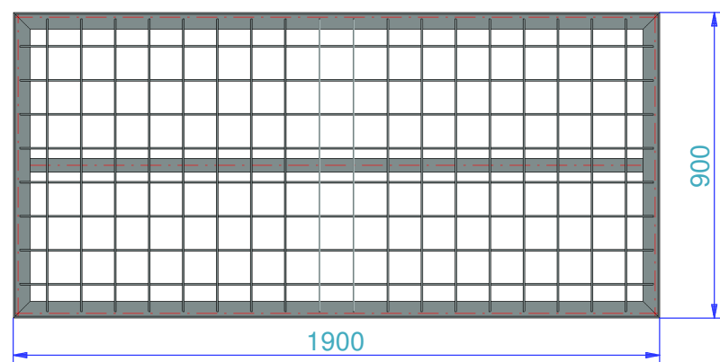
Einsatz mit Gitterrost zu Bett E190A
